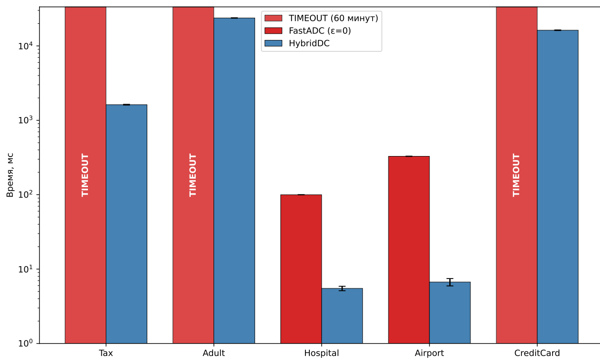
Рис. 8: Время перечисления покрытий: сравнение с FastADC при нулевом пороге ошибки.
