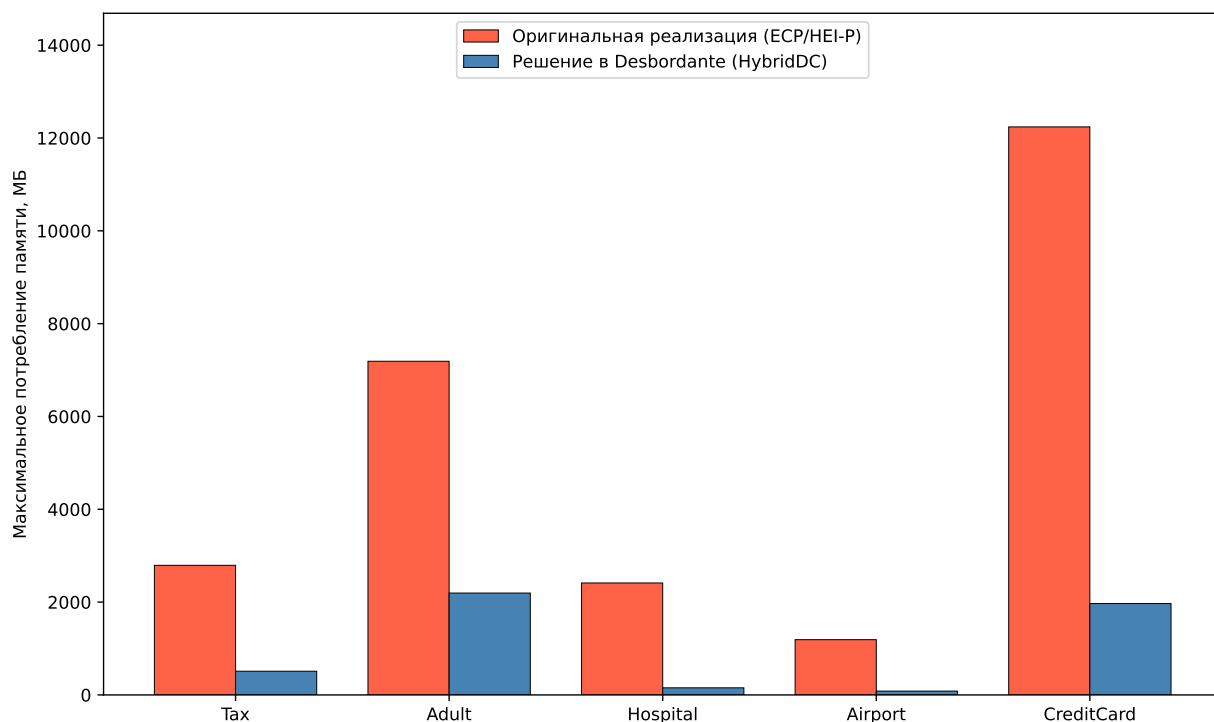
Рис. 7: Максимальное потребление памяти: сравнение с оригинальной реализацией.
