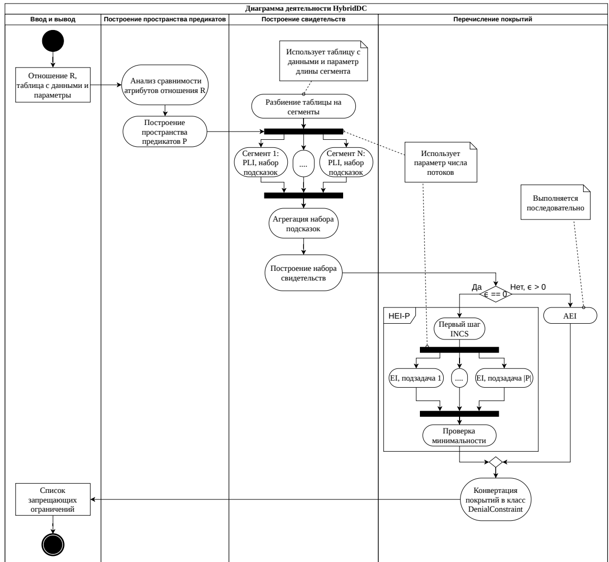
Рис. 2: UML-диаграмма деятельности, описывающая работу решения.
