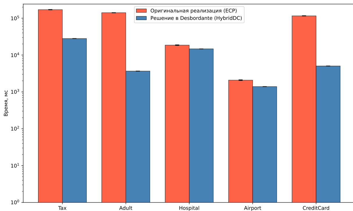
Рис. 4: Время построения набора свидетельств: сравнение с оригинальной реализацией.
