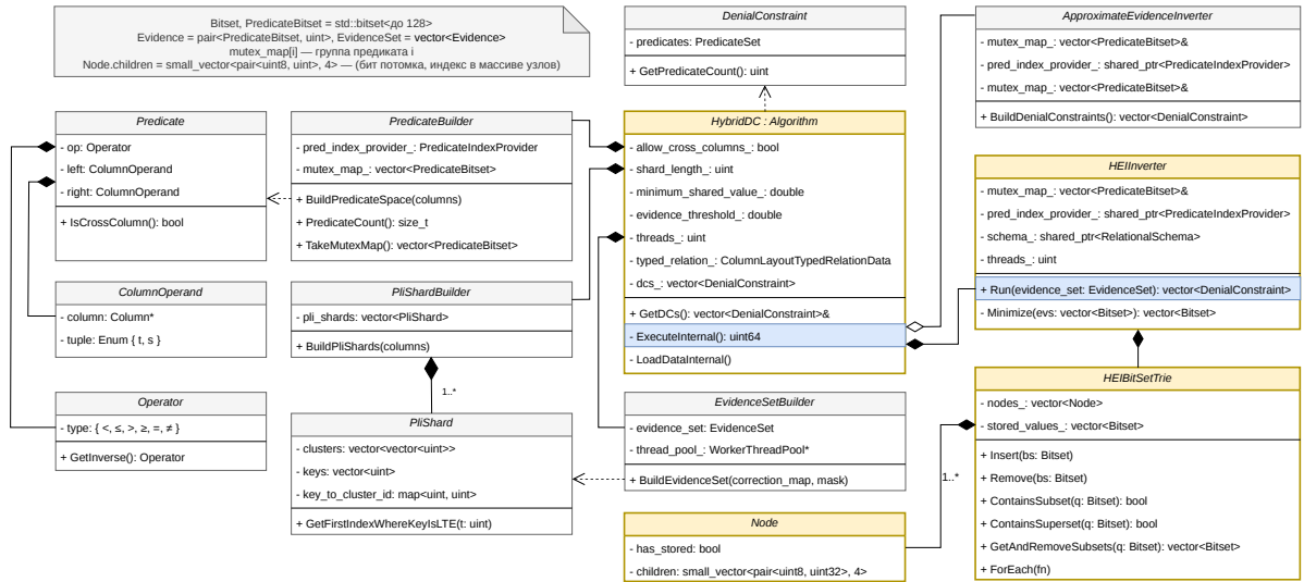
Рис. 3: UML-диаграмма классов алгоритма HybridDC.
