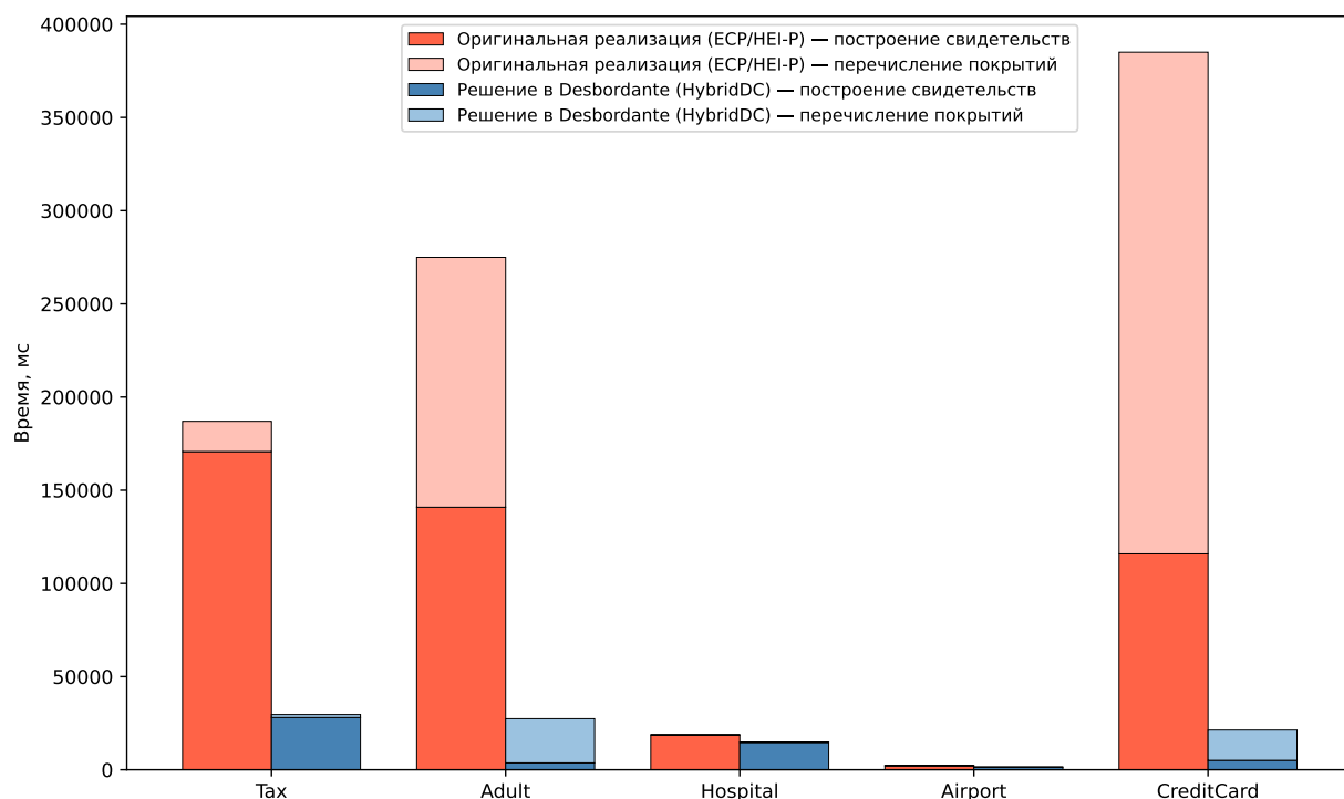
Рис. 6: Суммарное время выполнения: сравнение с оригинальной реализацией. Время представлено линейной шкалой. Каждая колонка разбита на два участка: нижний — время построения набора свидетельств, верхний — время перечисления покрытий.
