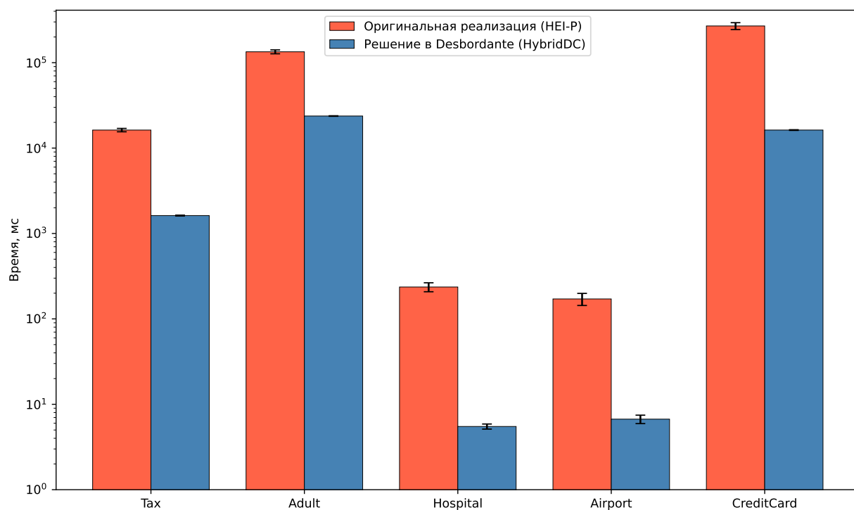
Рис. 5: Время перечисления покрытий: сравнение с оригинальной реализацией.
