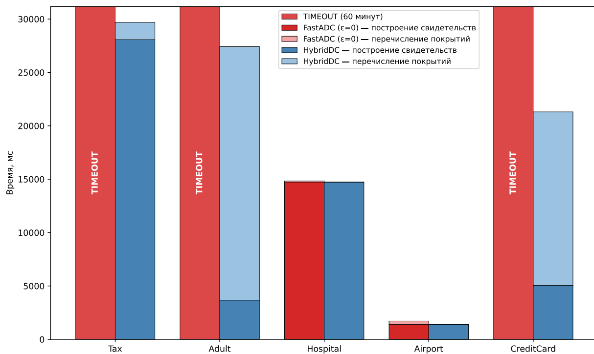
Рис. 9: Суммарное время выполнения: сравнение с FastADC при нулевом пороге ошибки. Время представлено линейной шкалой. Каждая колонка разбита на два участка: нижний — время построения набора свидетельств, верхний — время перечисления покрытий.
